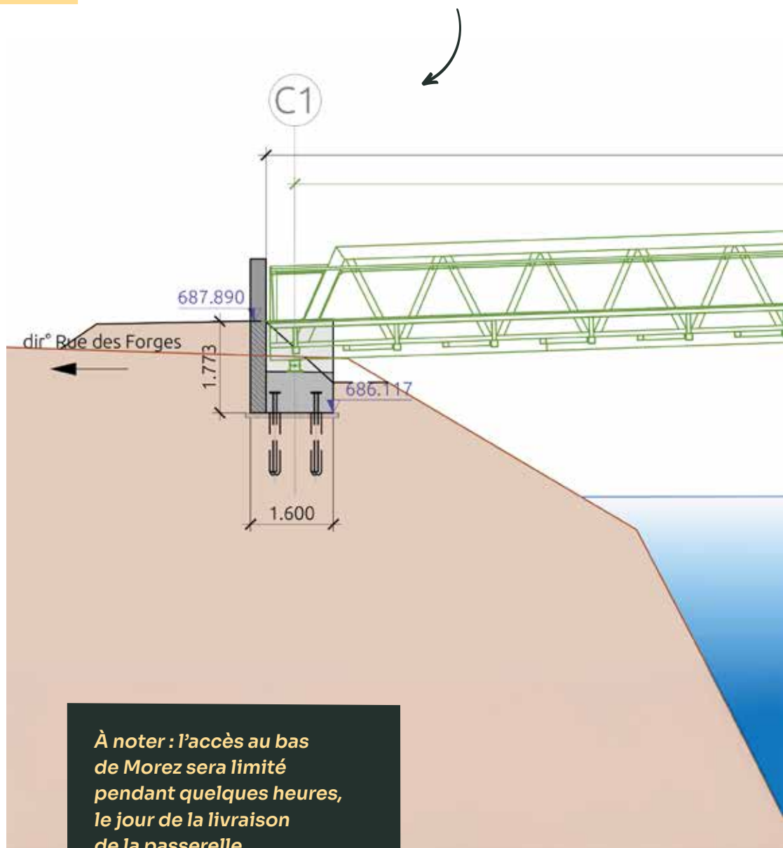
Plan technique de la future passerelle
